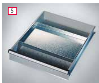
5 Schubfach-Einsatz Verschiebbar als zusätzliches Fach im Schubfach. Aus Stahlblech verzinkt.
