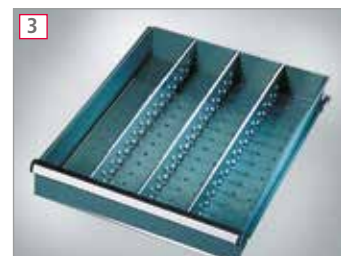
3 Sachschiene Aus Stahlblech verzinkt. Am Schubfachboden verschraubbar.
